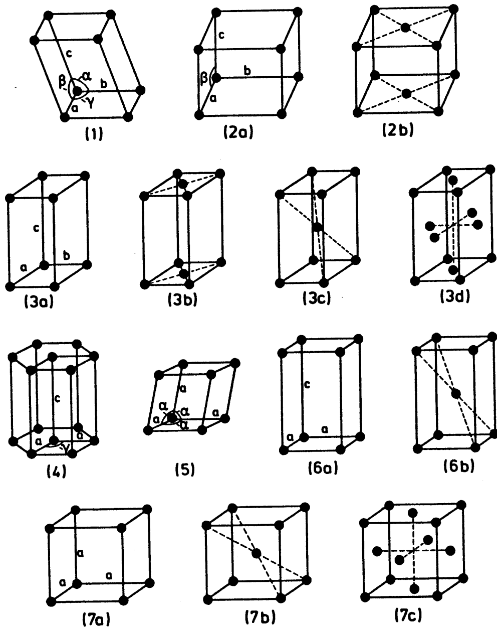
Abbildung 1.4: Die 14 Bravaisgitter: 1=triklin, 2=monoklin, 3=orthorhombisch, 4=hexagonal, 5=rhombisch, 6=tetragonal, 7=kubisch.
