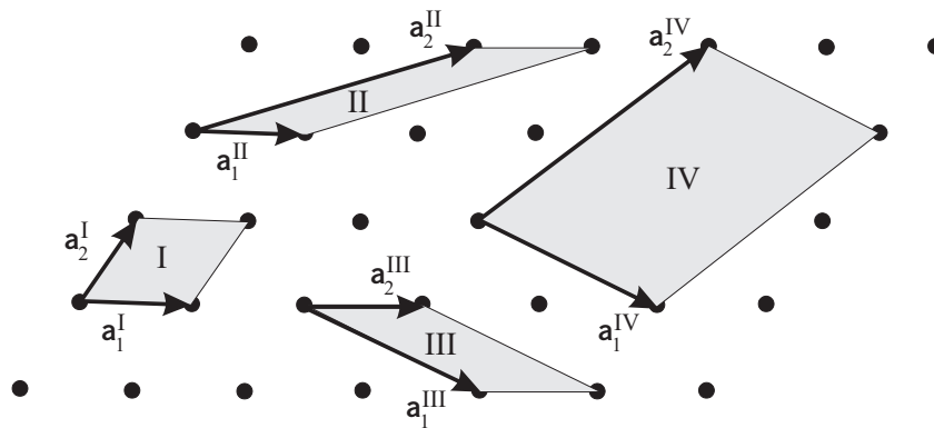
Abbildung 1.1: Skizze eines zweidimensionalen Raumgitters mit Gitterbausteinen.
